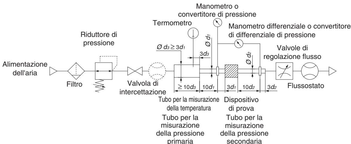
Fig. (1) Circuito di prova in conformità con ISO 6358:1989, JIS B 8390:2000
