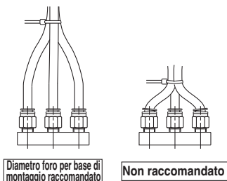
Fig. 2 Quando si utilizza una fascetta per unire le connessioni
