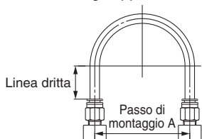
Fig. 1 Connessione raccomandata
